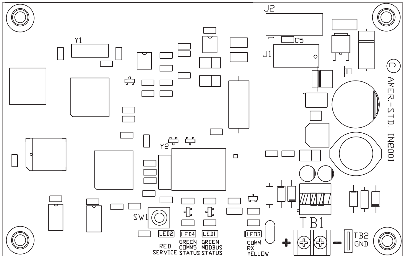
Figura 7 - Configuración de la interfaz de comunicación LCI-R LonTalk®
