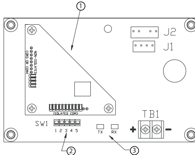
Figura 9 - Módulo de comunicaciones, configuración Tipo 1
