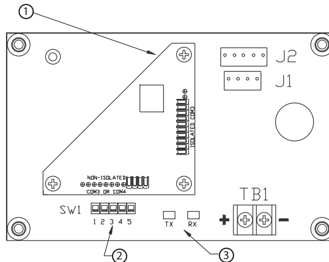
Figura 10 - Módulo de comunicaciones, configuración Tipo 2
