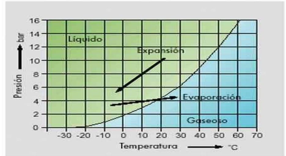
Curva de presión de vapor R134a
