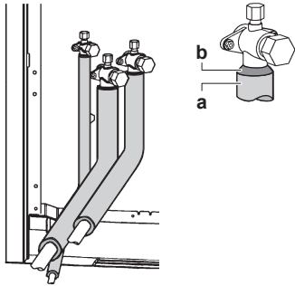
a Material de aislamiento b Calafateado, etc.
