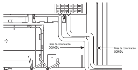
Conexión PCB principal
