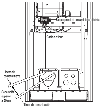
Conexión de suministro eléctrico principal
