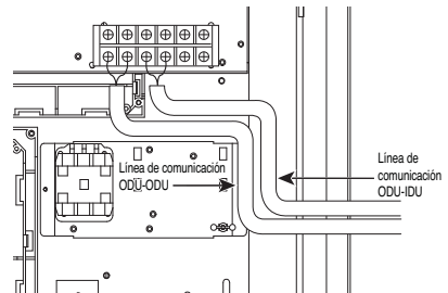
Conexión PCB principal
