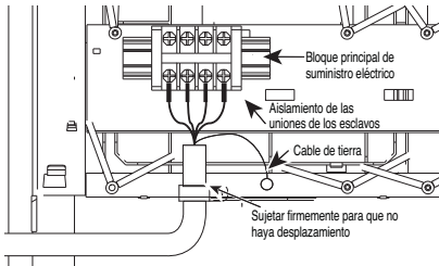
Conexión de suministro eléctrico principal
