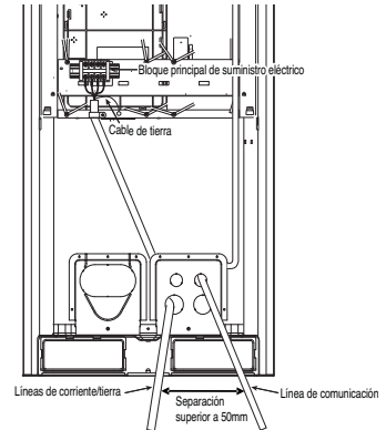
Conexión PCB principal
