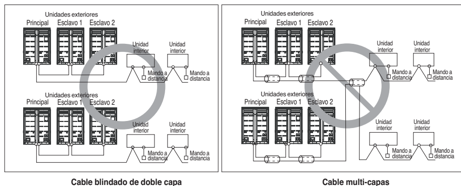
Cable blindado de doble capa
