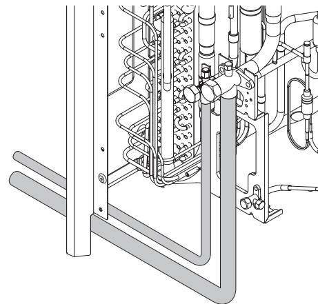
Retire solo la salida de líquido/gas
