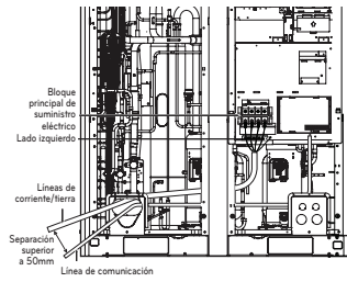
Conexión de suministro eléctrico principal
