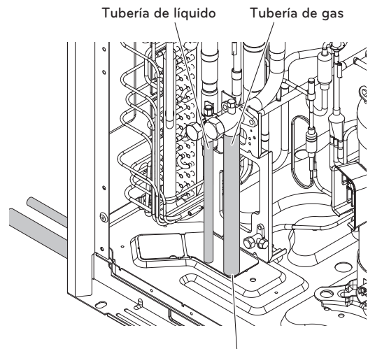
Retire solo la salida de líquido/gas
