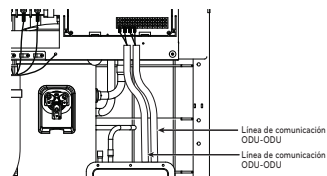
Conexión de comunicación
